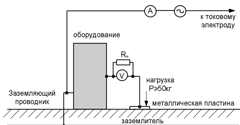
Рисунок 5 – Схема измерения напряжения прикосновения
