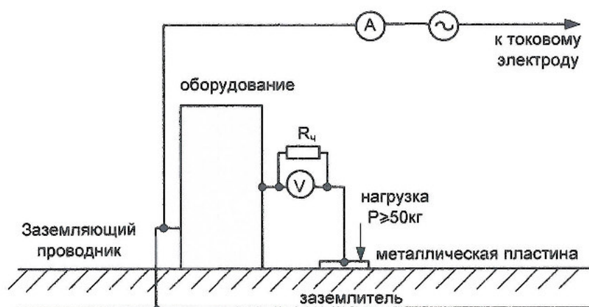
Рисунок 6 – Схема измерения напряжения прикосновения
