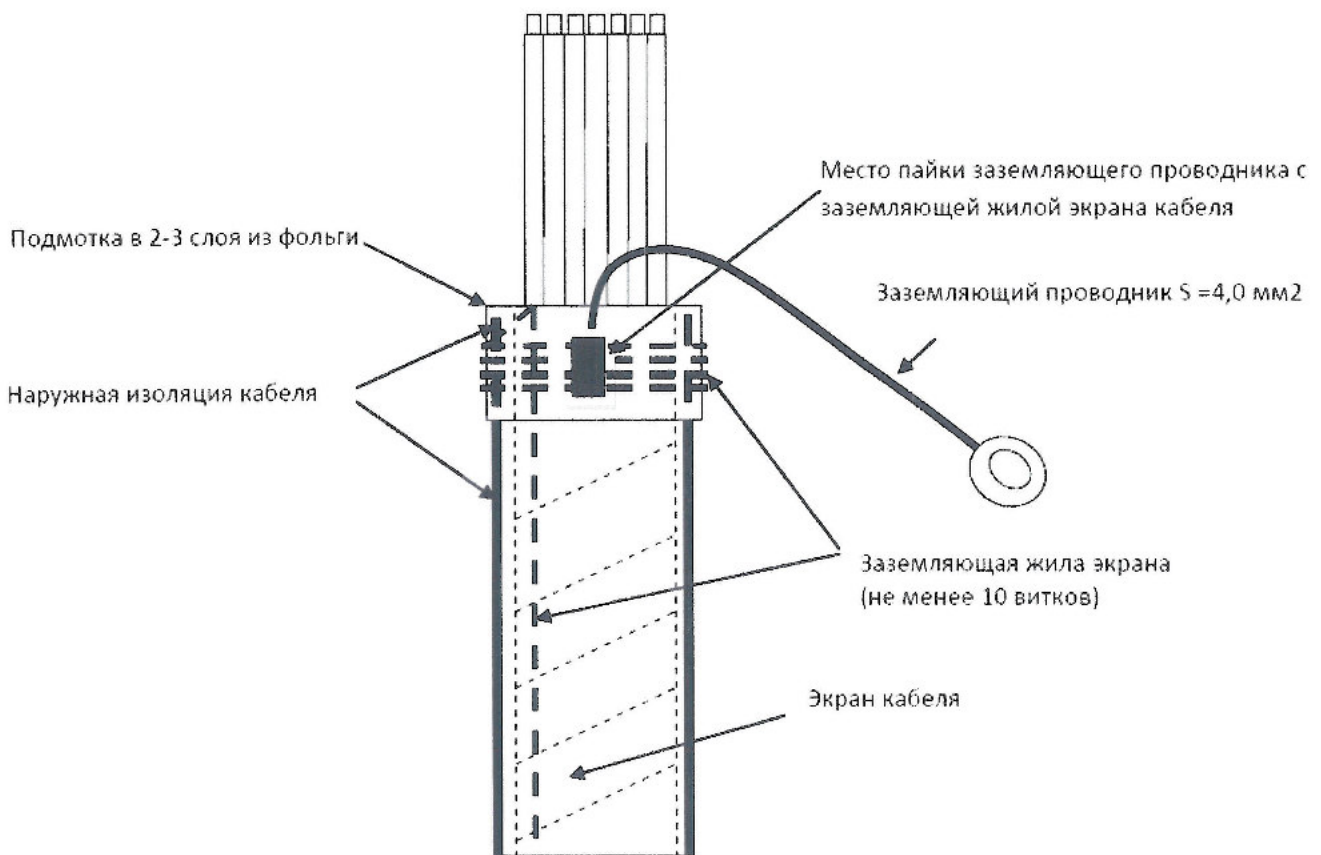
Рисунок 7 – Заземление экранов кабелей
