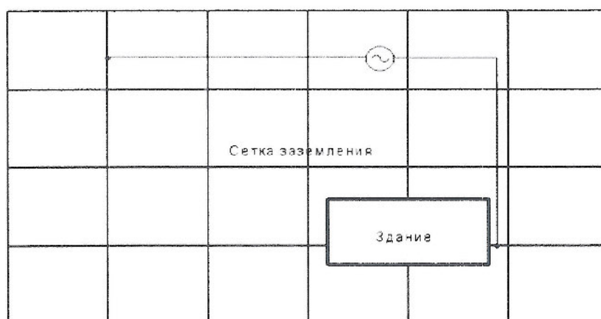
Рисунок 3 – Схема измерительной цепи при трассировке заземляющего устройства
