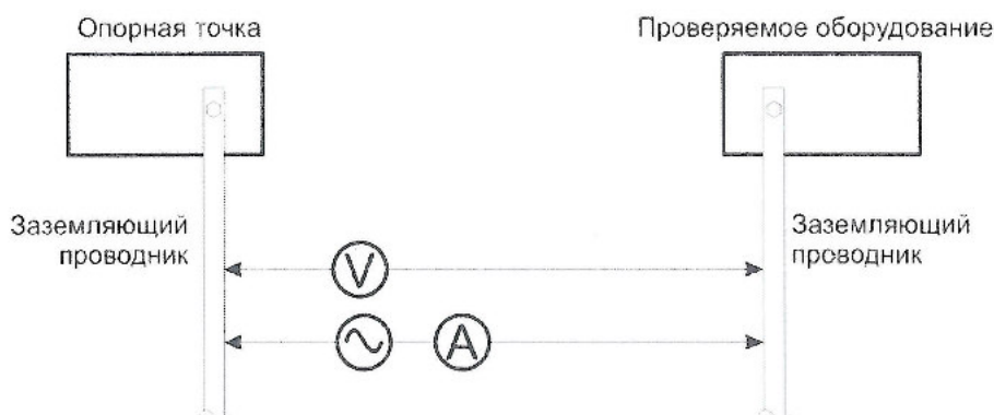
Рисунок 5 – Схема измерения сопротивления металлосвязи
